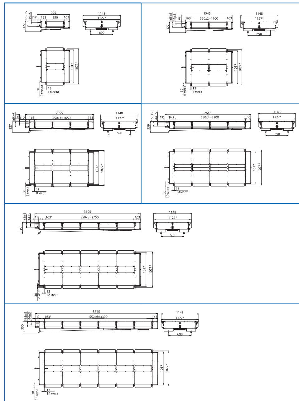
Габаритные и присоединительные размеры UDR.300
