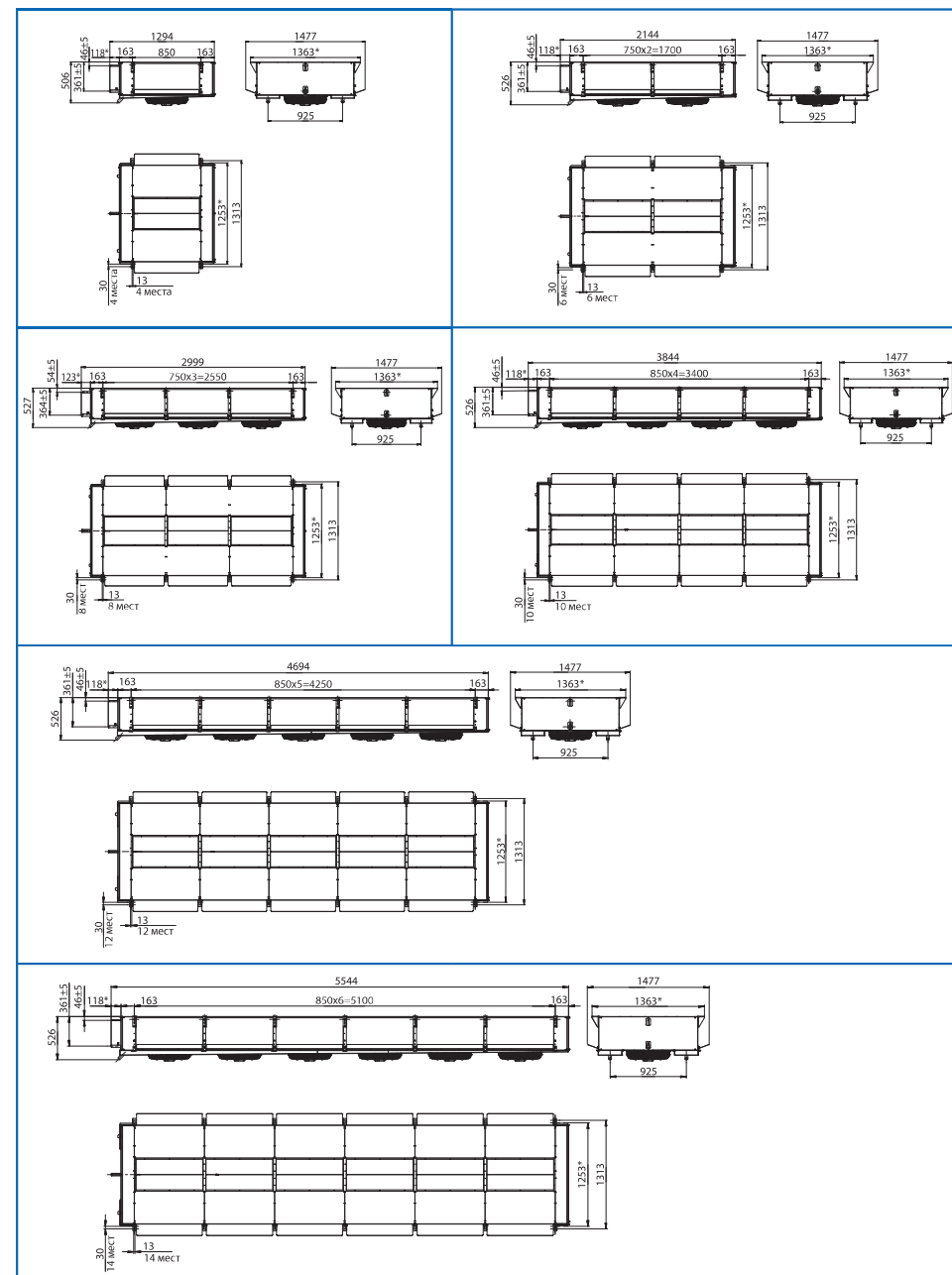
Габаритные и присоединительные размеры UDR.450
