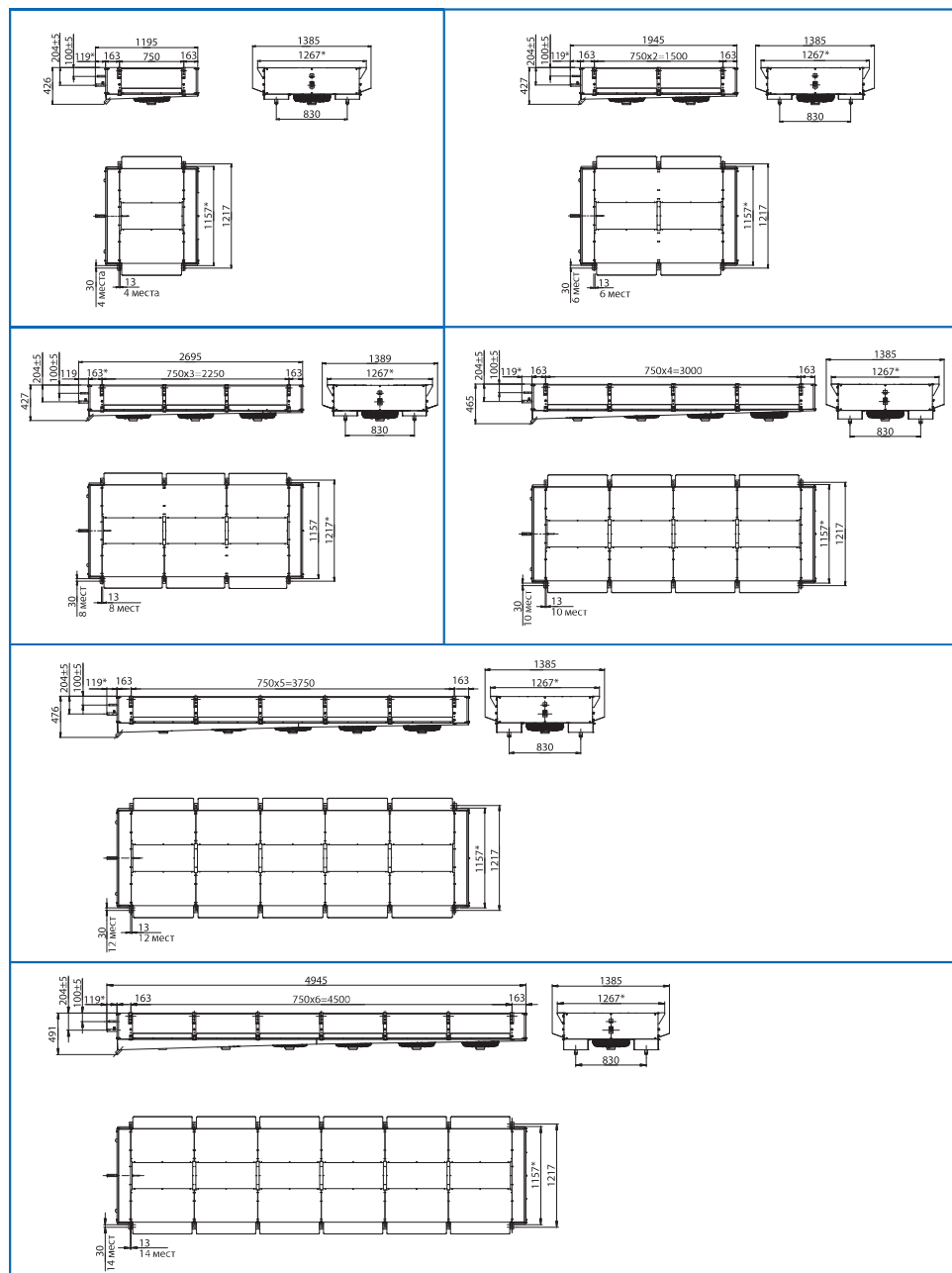
Габаритные и присоединительные размеры UDR.400
