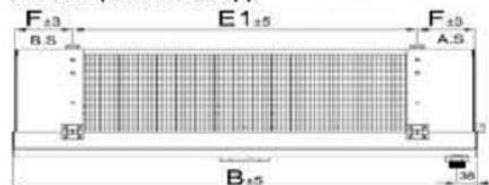
BS-TEM (1 вентилятор)
