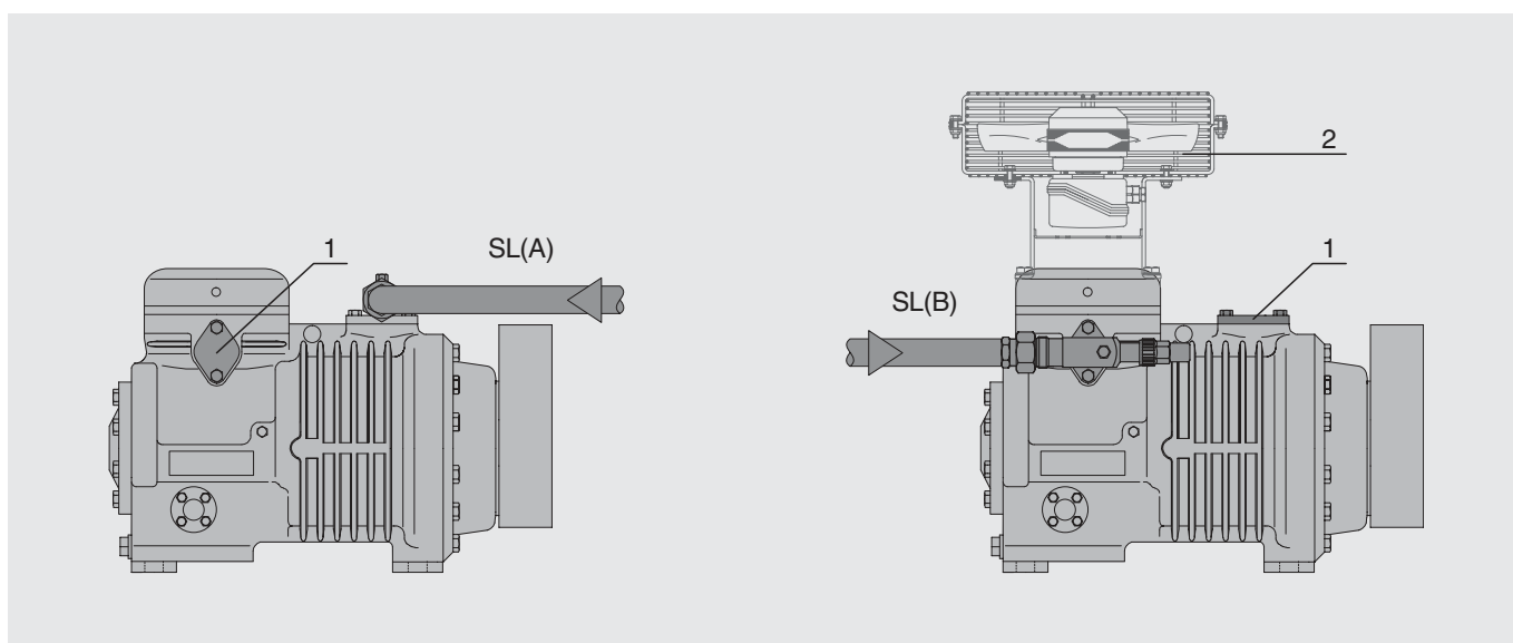
Abb. 5 VARICOOL-System SL(A) Sauggas-Kühlung SL(B) Direkt-Ansaugung 1 Blindflanssch 2 Zusatzlüfter alternativ: Aufstellung im Luftstrom des Verflüssigers
