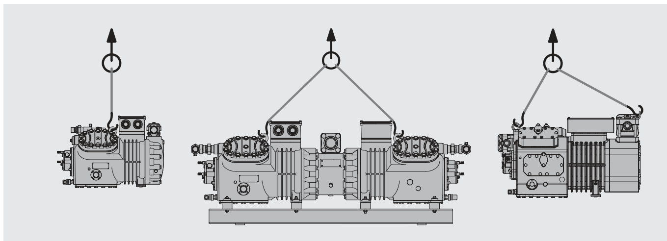
Abb. 1 Verdichter anheben
